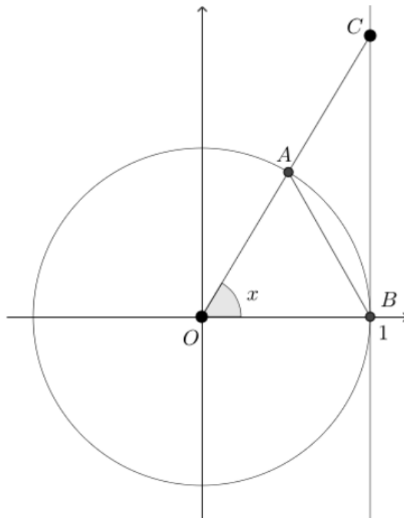
Рис. 3. Первый замечательный предел
